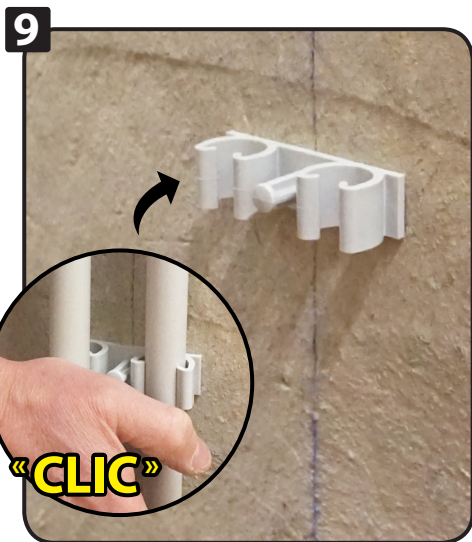
Clipsez les tubes à la main.
